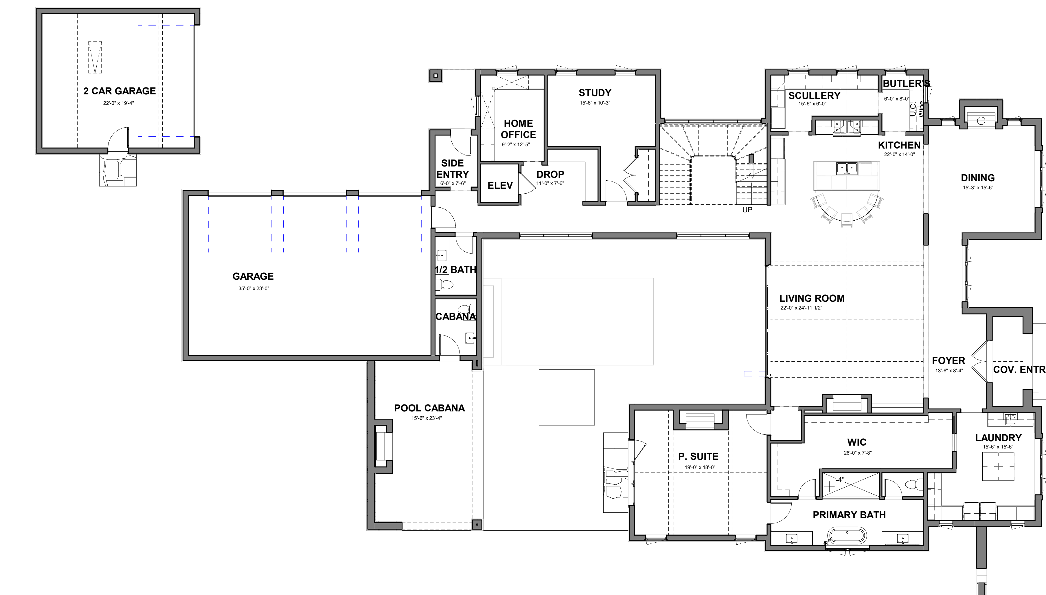
1 first floor scale: 1/8" = 1'-0"
